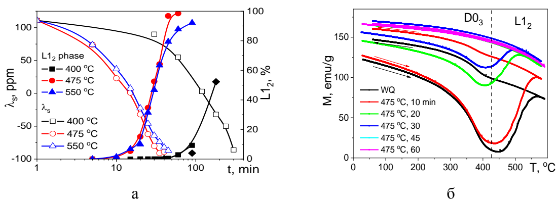
Рисунок 2. Графики зависимости изменения магнитострикции насыщения и доли фаз в сплаве Fe-27Ga от времени и температуры отжига (а) и температурной зависимости намагниченности от времени отжига (б)
