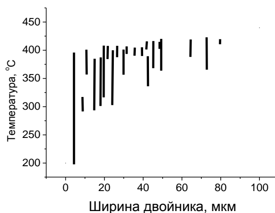
Рисунок 2. Зависимость величины температурного интервала движения НҚДГ от ширины двойников
