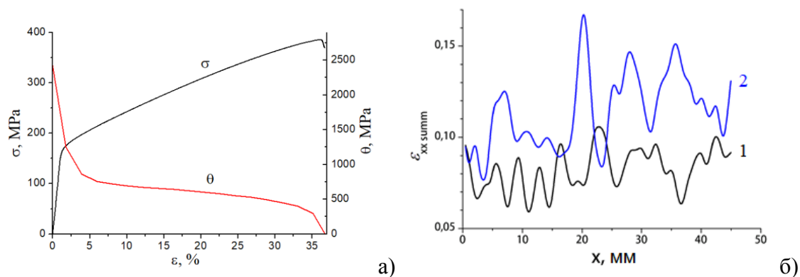
Рисунок 1. (а) Совмещенные зависимости напряжения \sigma и коэффициента деформационного упрочнения \theta от общей деформации \varepsilon ; (б) распределение накопления локальных деформаций вдоль оси растяжения в интервале \varepsilon=3-13\% (1) и \varepsilon=17-34\% (2)
