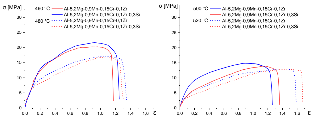
Рисунок 2 – Кривые деформации сплавов Al-5,2Mg-0,9Mn-0,15Cr-0,1Zr и Al-5,2Mg-0,9Mn-0,15Cr-0,1Zr-0,3Si с постоянной скоростью 2 \times 10^{-3} \text{ c}^{-1}
