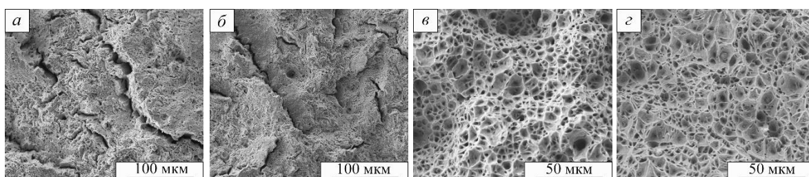
Рисунок 2. Фрактограммы образцов стали ЭК-181 после ТТО (а, в) и «ТТО + выдержка в жидком свинце» (б, г), после растяжения при 20 °С (а, б) и 720 °С (в, г)
