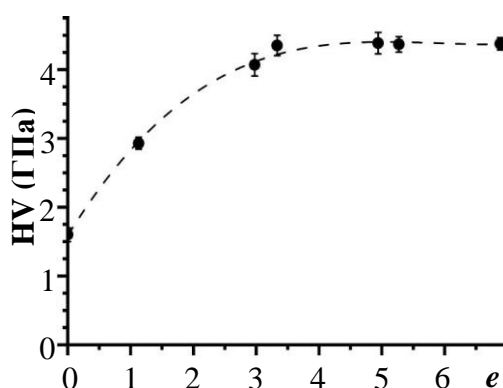
Рисунок 1. Зависимость микротвердости сплава V-Cr-W-Zr от степени деформации
