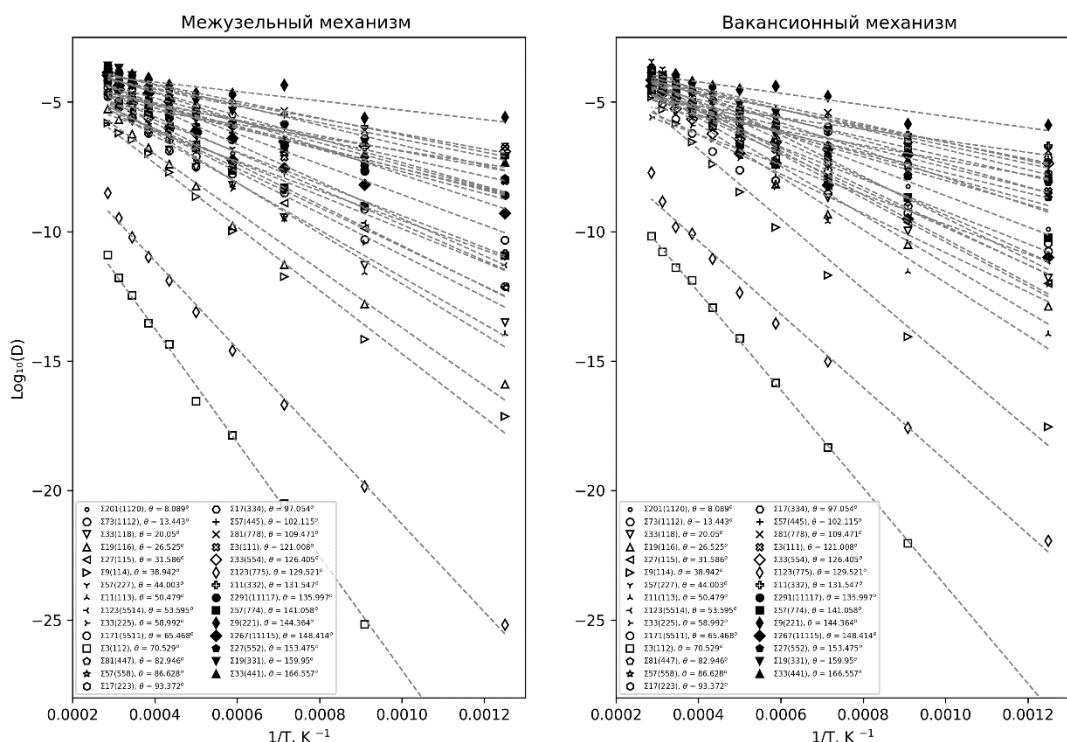
Рисунок 2. Температурные зависимости коэффициентов зернограничной самодиффузии в границах зерен наклона \langle 110 \rangle в вольфраме для вакансионного и межузельного механизмов.
