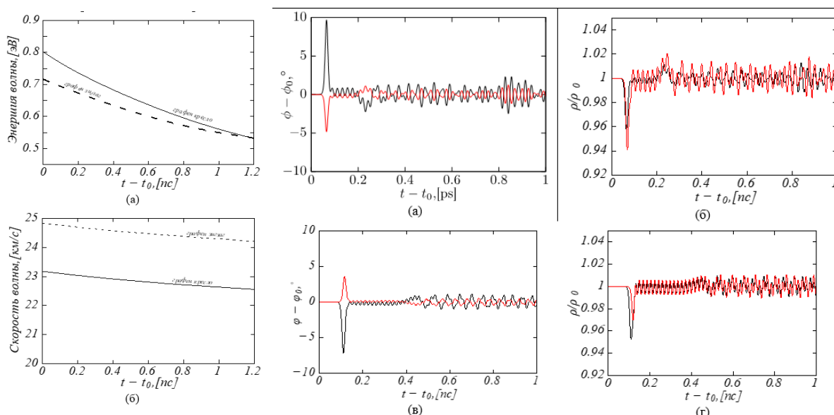
Рисунок 1. (Слева) Эволюция энергии (а) и скорости солитона (б) во времени для E_0 - E_{rest} . Сплошная линия для направления кресло, штрихованная - зигзага. T_0 = 1 пс. (Справа) Динамика угла \phi и длины r связи во времени при прохождении через атомы солитонной волны. Черный цвет кривых зависимостей соответствует углу \phi_1 и длине r_1 , красный – углу \phi_2 и длине r_2 . Левые графики соответствуют зависимостям \phi(t) - \phi_0 , а правые – r/r_0(t) . (а) и (б) - графен, направление кресло, (в) и (г) - графен, направление зигзаг
