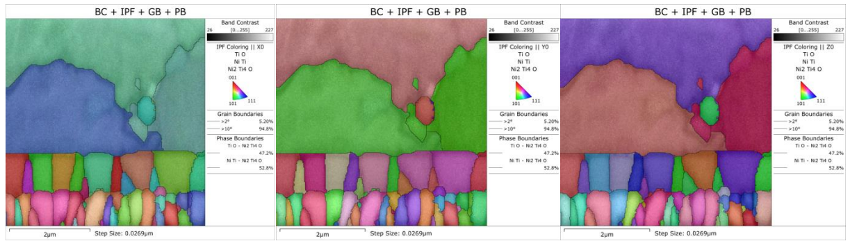
Рисунок 1. EBSD анализ микроструктуры эквиатомного никелида титана с композитным покрытием. Ориентационные карты в цветах полюсных фигур.
