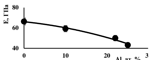
Рисунок 1 Зависимость модуля упругости сплавов системы Ni_{50}Mn_{50-y}Al_y
