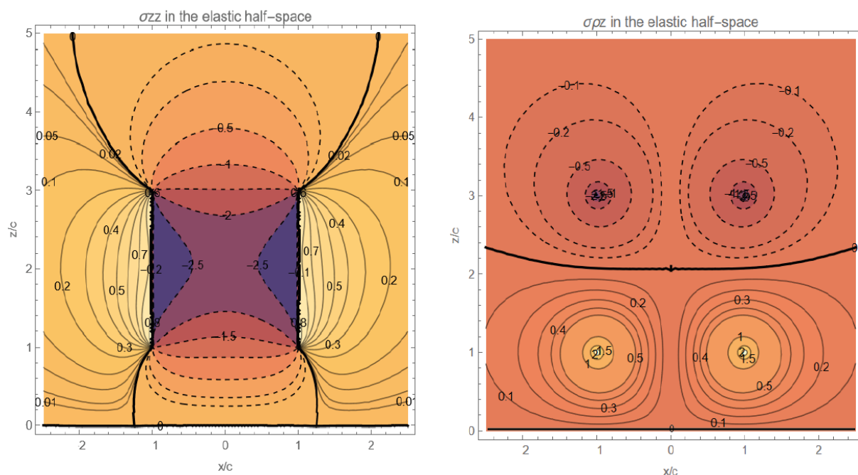
Рисунок 2. Карты напряжений \sigma_{zz} и \sigma_{rz} в центральном продольном сечении цилиндрического включения в упругом полупространстве. Координата свободной поверхности: z = 0 . Напряжения выражены в единицах G\varepsilon^* , где G – модуль сдвига, \varepsilon^* – величина собственной деформации включения. В расчетах коэффициент Пуассона \nu = 0.3 . Координаты нормированы на величину радиуса цилиндра s .
