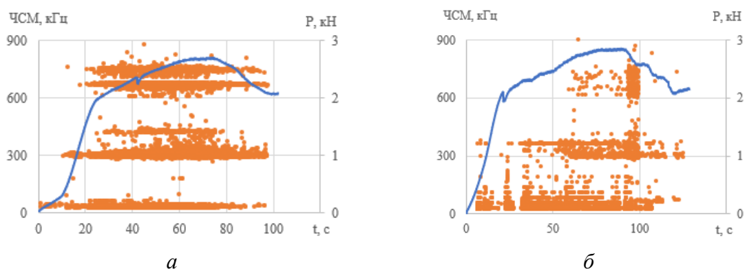
Рисунок 2. Диаграммы зависимости пиковых амплитуд сигналов АЭ от времени, совмещенные с графиком нагружения образцов без дефектов (а) и образцов с непроклеем (б)
