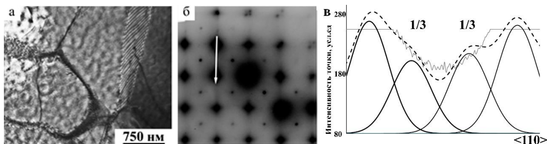
Рис. 1. Светлопольное изображение (а), микроэлектронограмма (б, ось зоны [001]_{B2} ) и профиль сканирования интенсивностей тяжей в направлении \langle 110 \rangle (в) микроструктуры сплава Ni_{50}Mn_{30}Al_{20}
