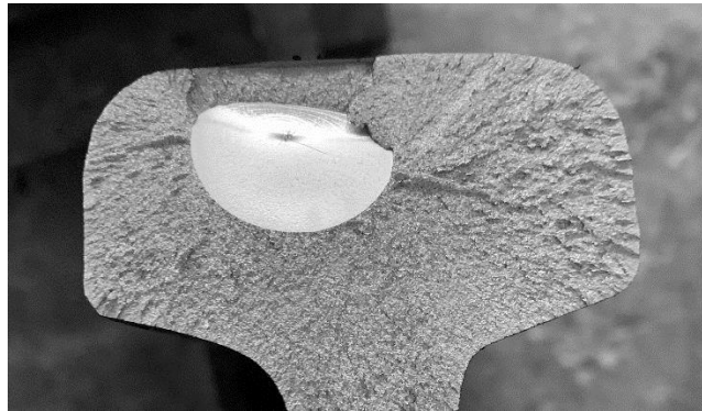
Рис.1. Внутренняя поперечная трещина в головке рельса
