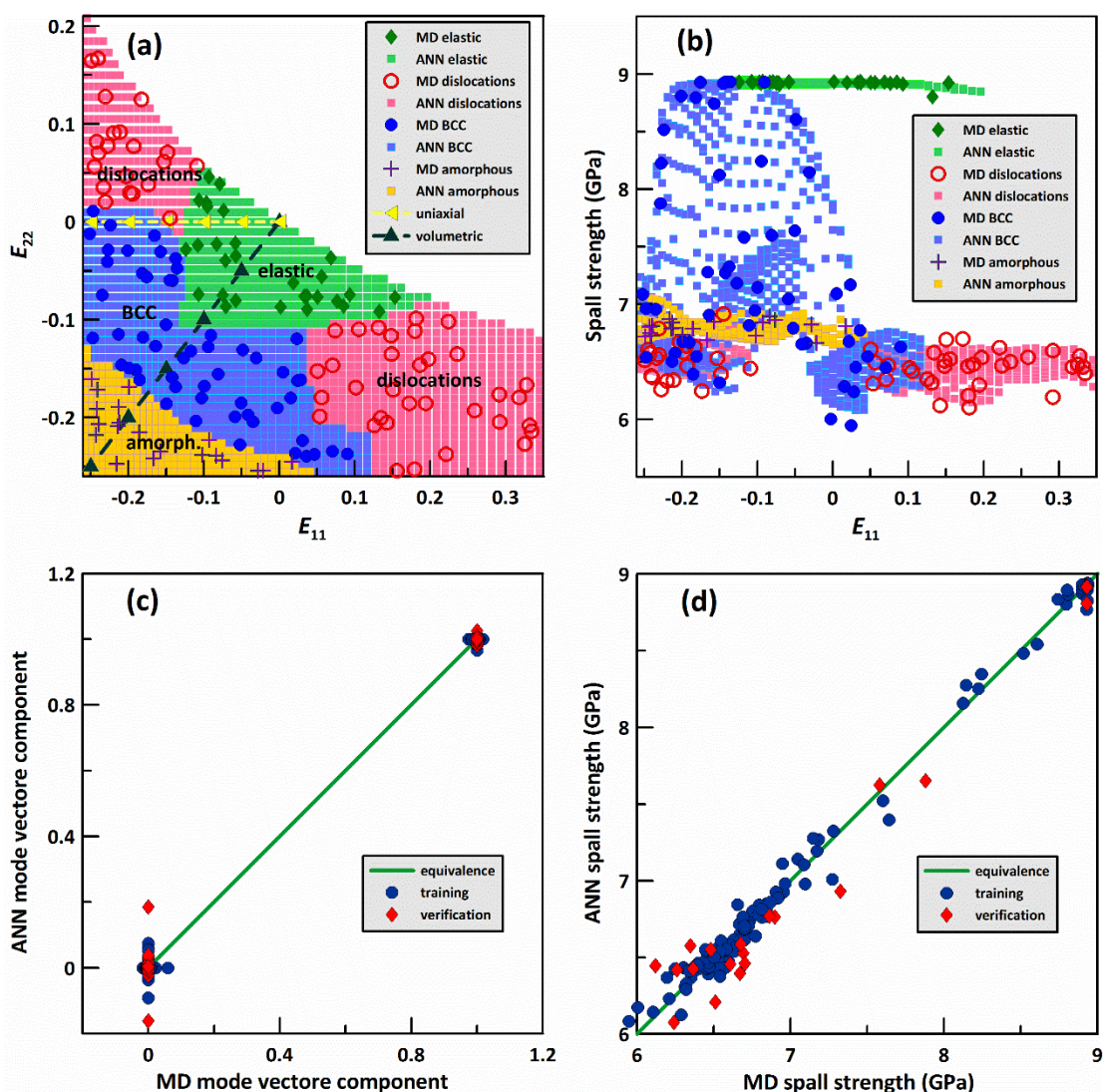
Рисунок 1. Зависимость откольной прочности алюминия от предварительной деформации [1] – анализ данных МД при помощи ИНС: (a) классификация деформированных состояний монокристалла (упругая область, дислокационная пластичность, фазовые переходы), (b) откольная прочность для разных предварительно деформированных состояний и (c,d) корреляционные графики обученных ИНС.
