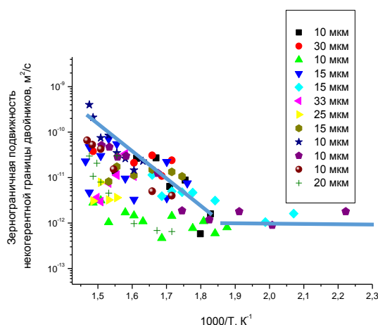
Рисунок 1. Температурная зависимость подвижности НҚДГ для двойников разной ширины
