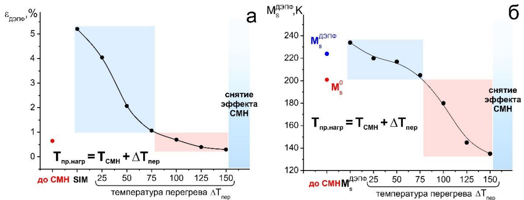
Рисунок 2. Термическая стабильность в монокристаллах Ni_{44}Fe_{19}Ga_{27}Co_{10} на параметры ДЭПФ \epsilon_{ДЭПФ} (а) и M_s^{ДЭПФ} (б)
